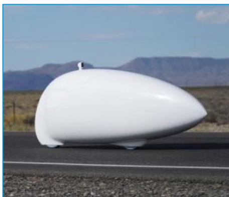
Vélo caréné couché Altaïr, Battle Mountain – 09/2022
